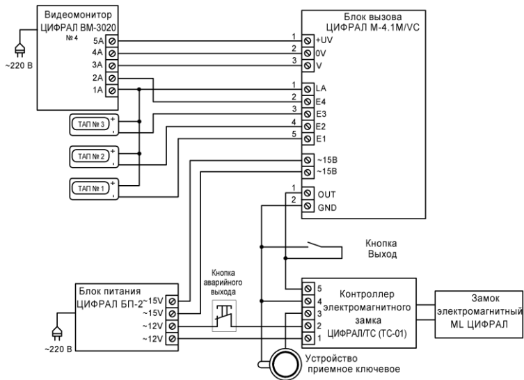
Рисунок Б.3 Схема подключения домофонов ЦИФРАЛ М-4.1М/ВС
