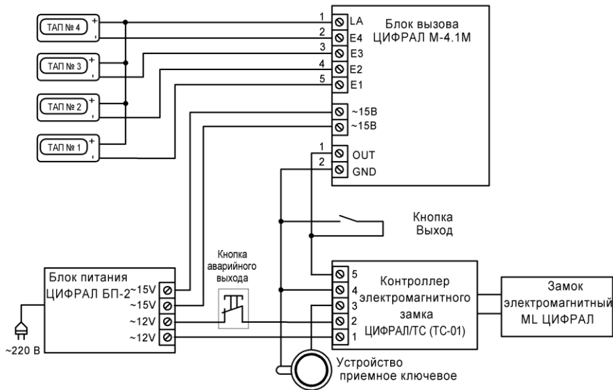
Рисунок Б.2 Схема подключения домофона ЦИФРАЛ М-4.1М
